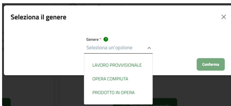
Figura 44: Voce composta
