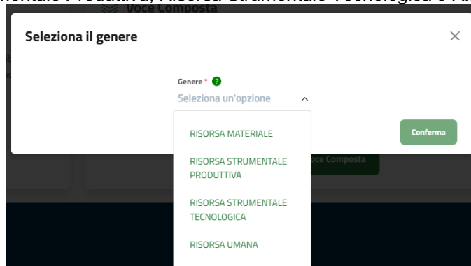
Figura 42: Voce semplice
