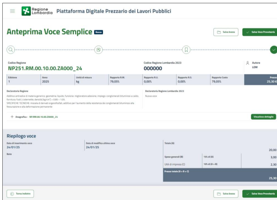
Figura 41: Anteprima Voce
