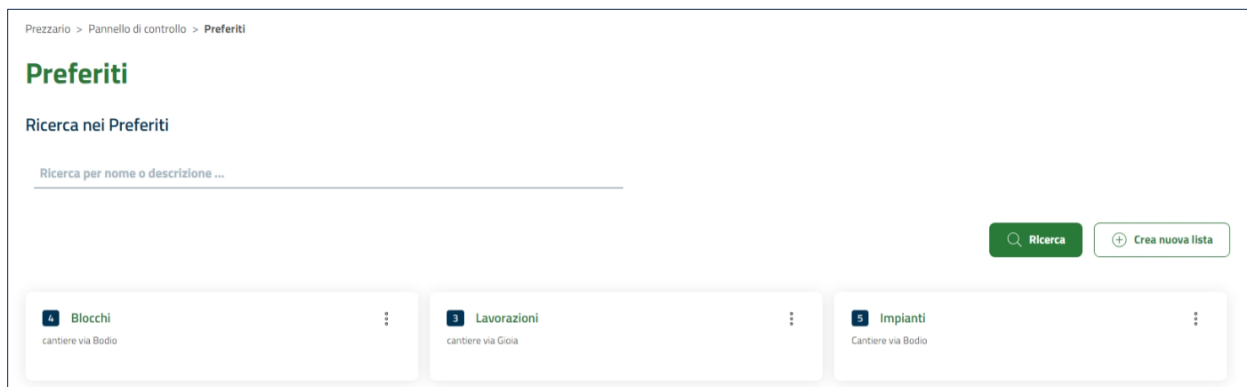
Figura 23: Lista preferiti
