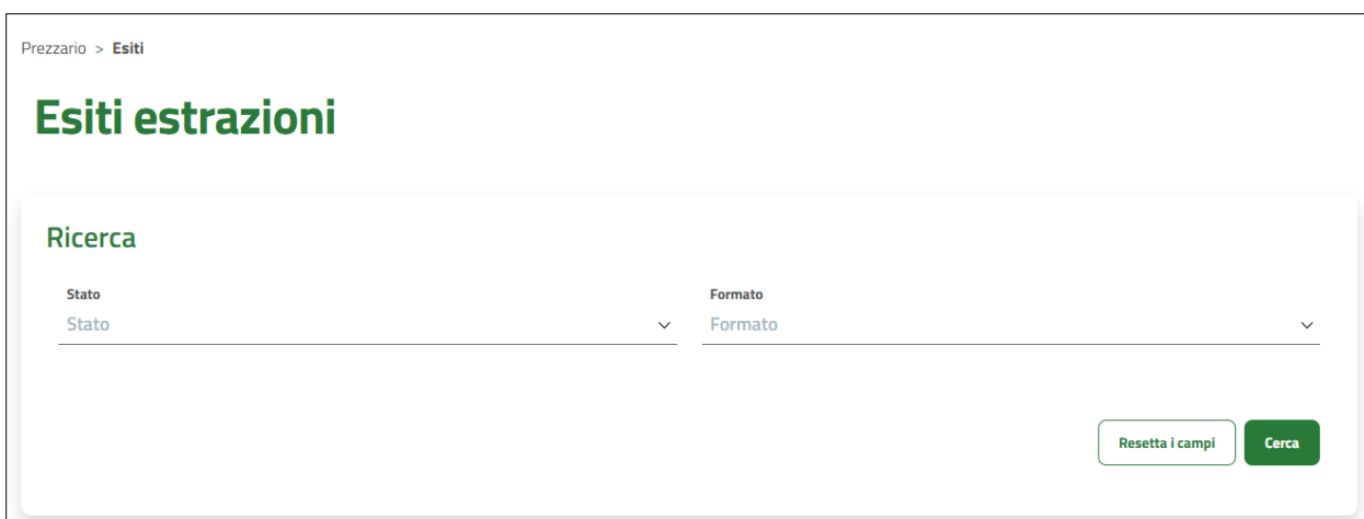
Figura 11: Esiti estrazioni
