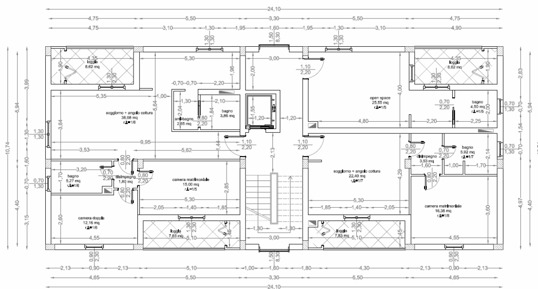
FIGURA 4. – PIANO TIPO del fabbricato residenziale.
